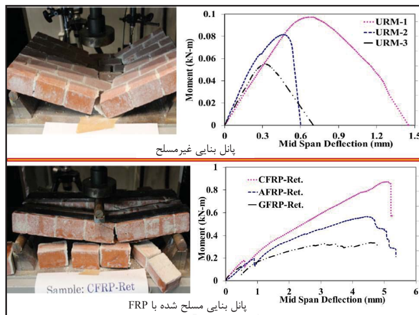
شکل ۱-۱۵- مسطح کردن المان بنایی با استفاده از FRP برای بهبود رفتار خمشی [۲۲]
